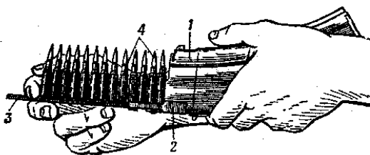
Снаряжение магазина патронами из обоймы: 1 - магазин; 2 - переходник; 3 - обойма; 4 - патроны
